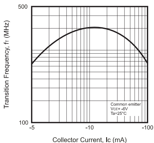
Fig.5 - f_T - I_c
